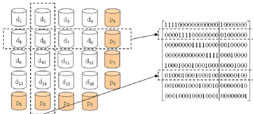
图 1 二维阵列编码及校验矩阵
